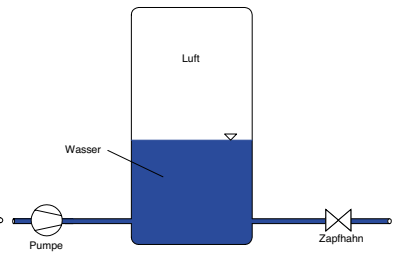
Verzinkter Windkessel
