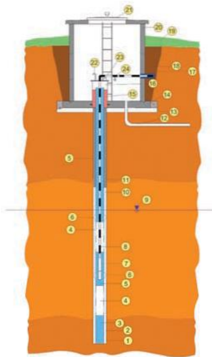
Schemazeichnung OÖ WASSER
