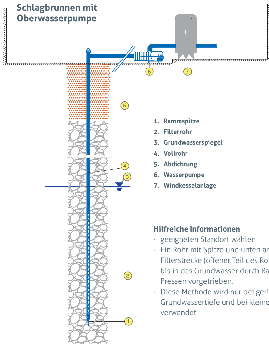
Schemazeichnung OÖ WASSER
