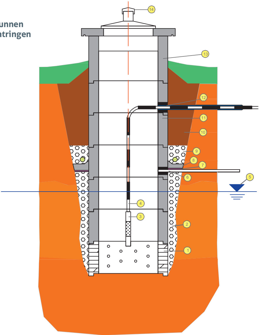
Schemazeichnung OÖ WASSER
