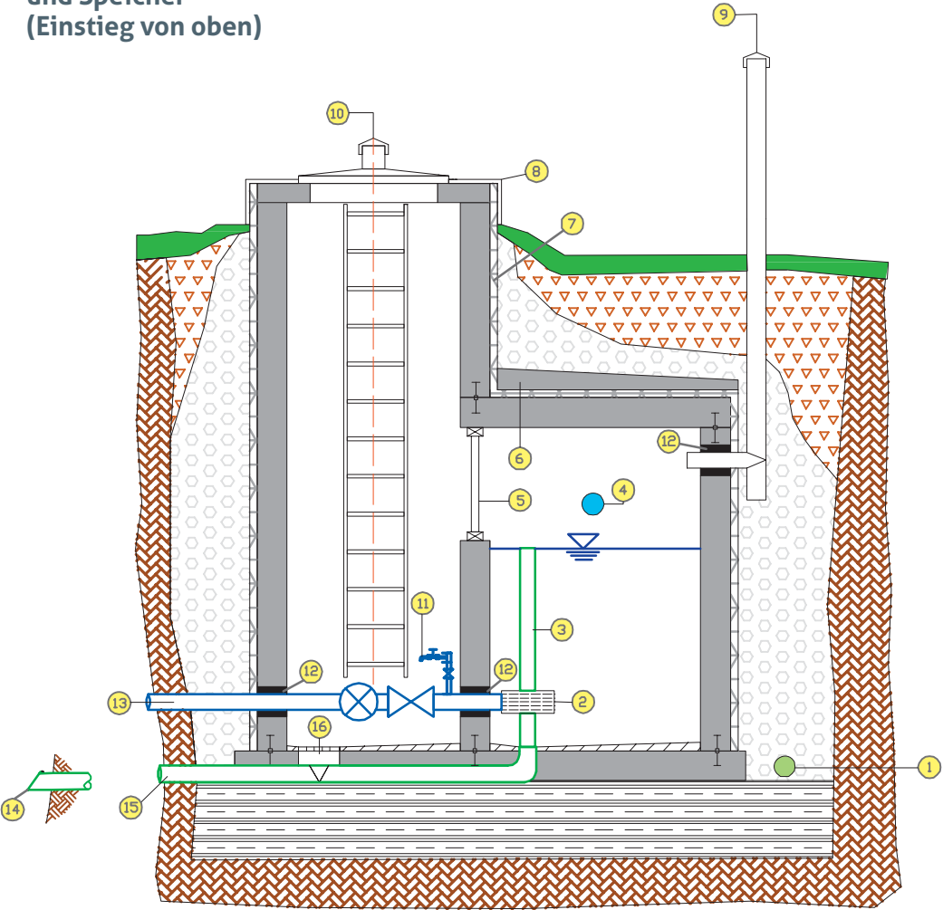
Schemazeichnung OÖ WASSER
